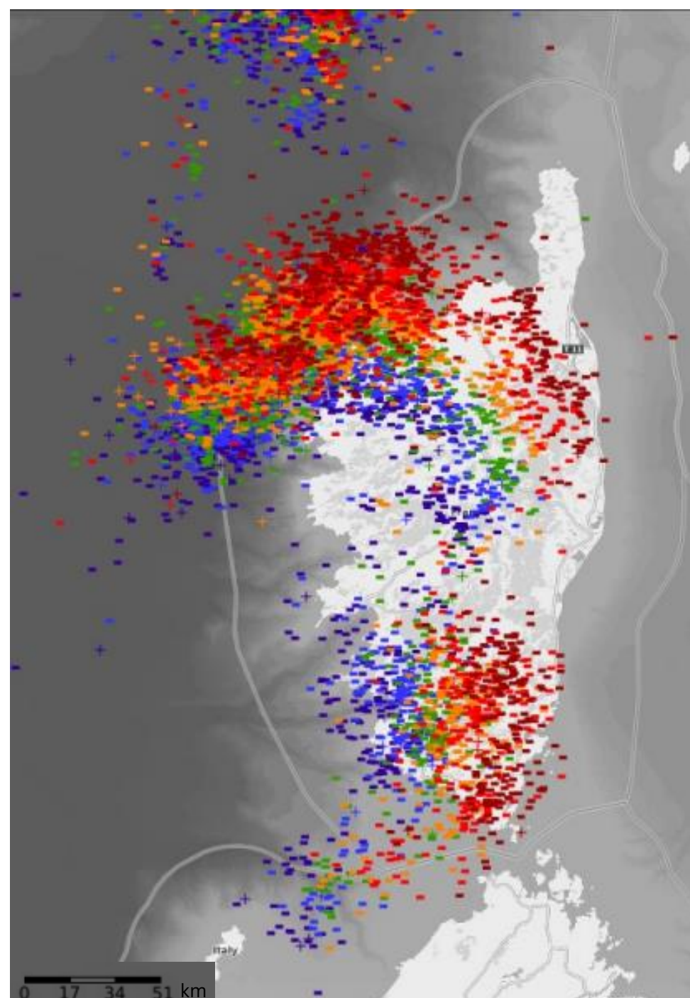
Activité foudre (éclairs nuage-sol CG) sur la zone de la Corse (maritime et terrestre) le 18 août 2022 entre 8h30 et 9h00
